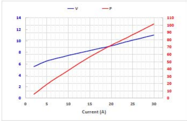
Fig.1 峰值功率 VS 正向电压 VS 正向电流 T_A = 25\text{ }^\circ\text{C}
