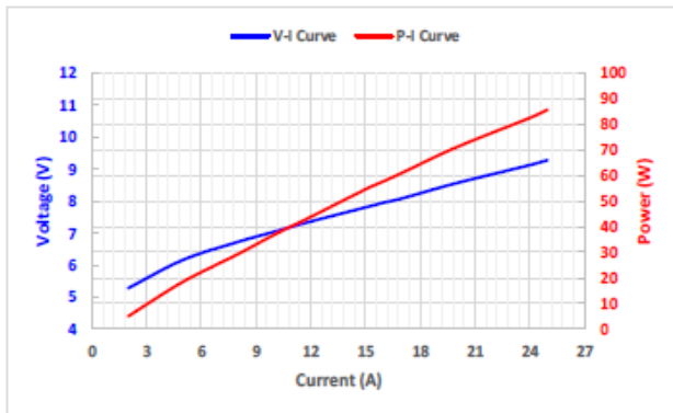
Fig.1 峰值功率 VS 正向电压 VS 正向电流 T_A = 25\text{ }^\circ\text{C}
